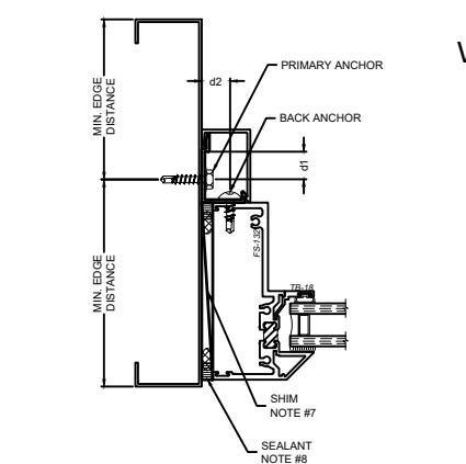
JAMBS
